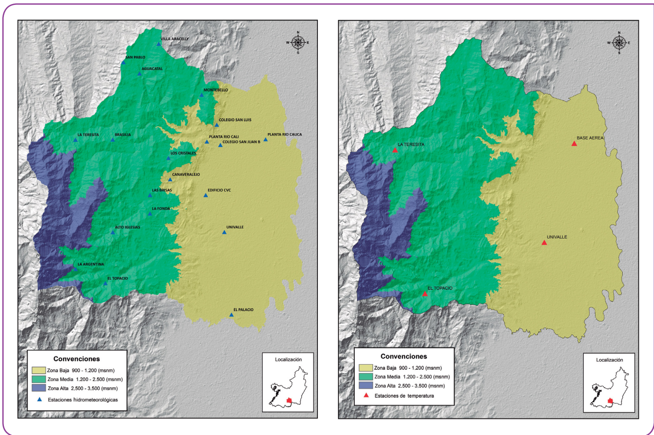
Figura 8. Zonificación altitudinal de las estaciones de precipitación (izquierda) y temperatura (derecha).
