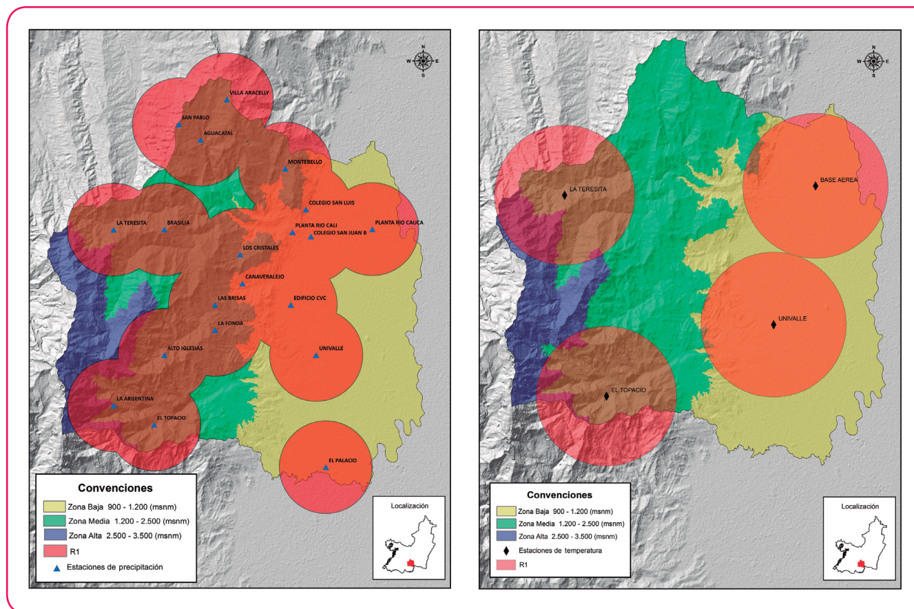
Figura 9. Radio de influencia de las estaciones de precipitación (izquierda) y temperatura (derecha).
