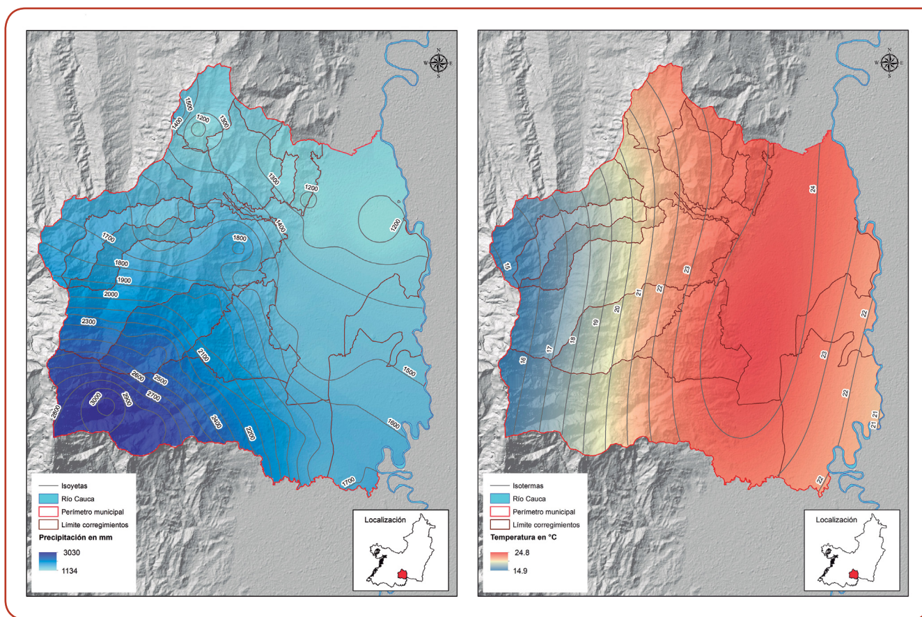
Figura 3. Isoyetas e isotermas medias anuales multianuales.
