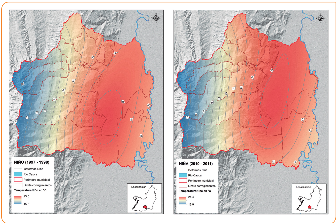
Figura 7. Isothermas eventos extremos ENOS (°C).
