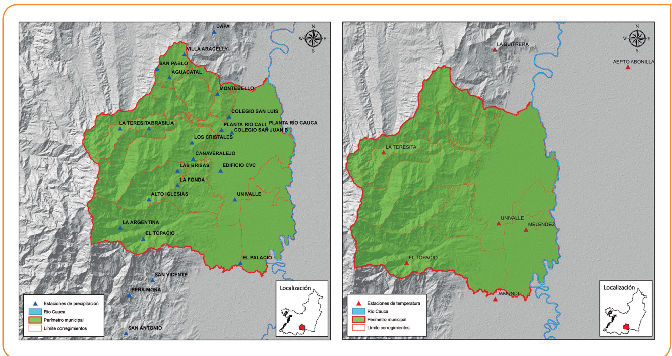
Figura 2. Ubicación de las estaciones de precipitación (izquierda) y temperatura (derecha) analizadas.
